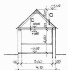
3-3 METSZET M=1:100
