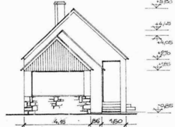
D. - NY. - I HOMLOKZAT M=1:100
