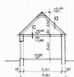
2-2 METSZET M=1:100
